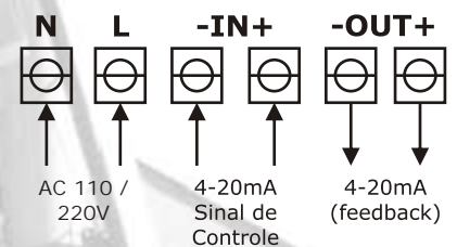
ESQUEMA ELÉTRICO DE LIGAÇÕES
